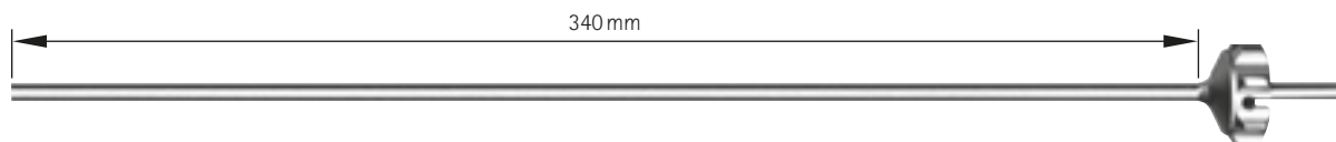
Schaft für bipolare Koagulationszange, Länge 340 mm, Ø 5 mm Shaft for bipolar coagulation grasping forceps, length 340 mm, Ø 5 mm
